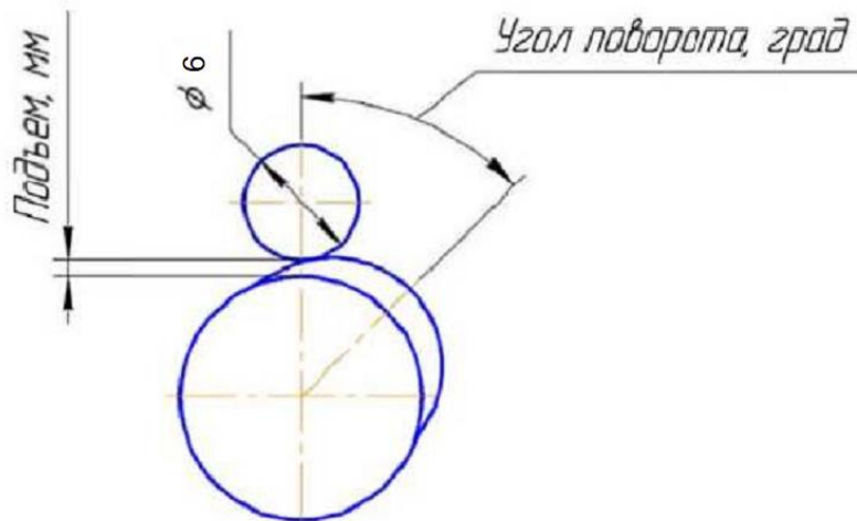
Схема измерения профиля кулачка
